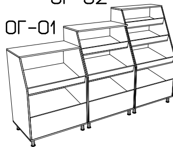
комплект горок
