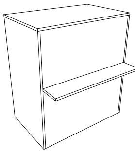
стол рабочий широкий (с полкой) 900x800x500
