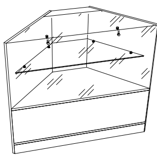
прилавок угловой наружный 900x700x700x500
